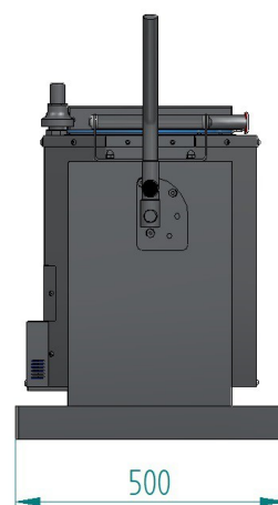
SEITENANSICHT
