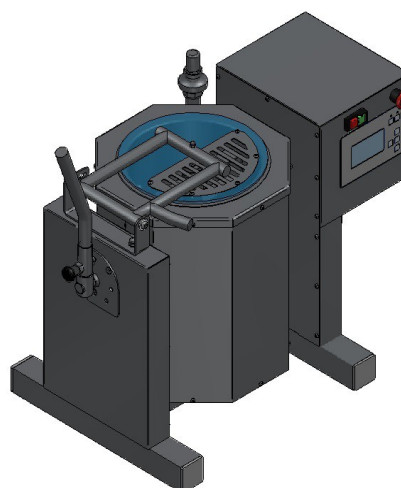
ISOMETRISCHE ANSICHT
