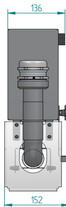
VISTA PLANTA
