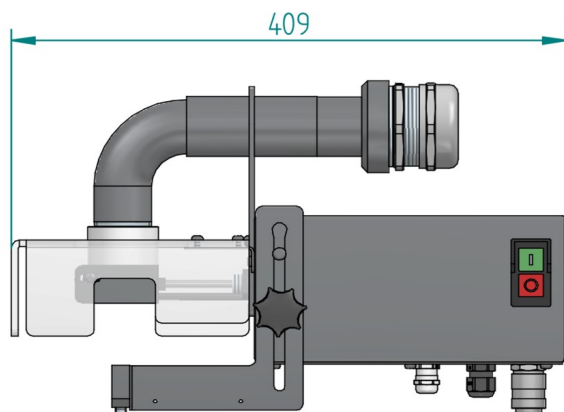
VISTA LATERAL
