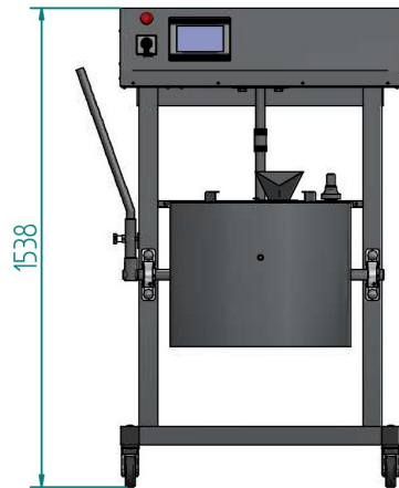
FRONTANSICHT
