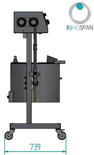
VISTA LATERAL
