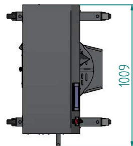
GRAUFSICHT
