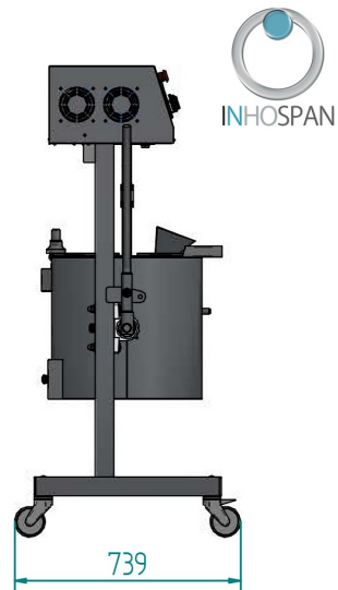
SEITENANSICHT
