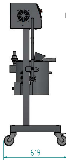
SEITENANSICHT
