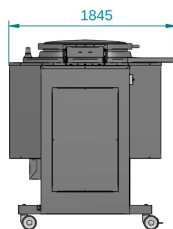
VISTA LATERAL
