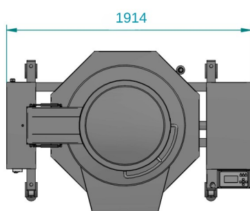
VISTA PLANTA
