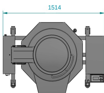
VISTA PLANTA
