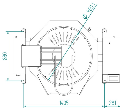
VISTA PLANTA
