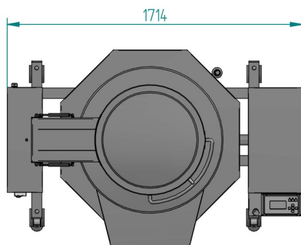
VISTA PLANTA
