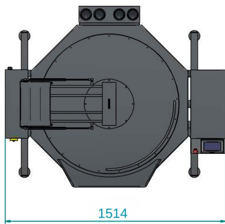
VISTA PLANTA
