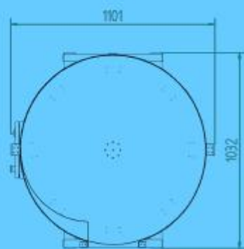
VISTA PLANTA
