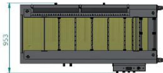
VISTA PLANTA
