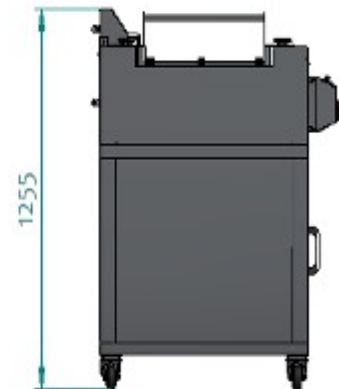
SEITENANSICHT
