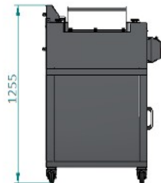
SEITENANSICHT
